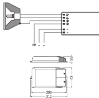
Technische Daten Osram PTi 150/220-240 I
